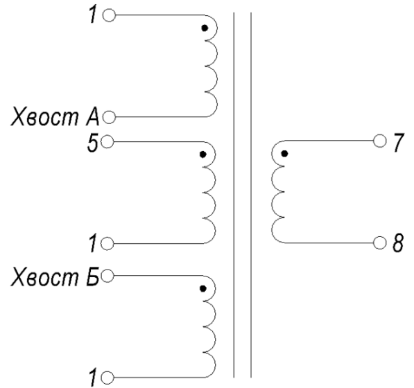
Электрическая схема
