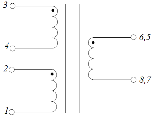
Электрическая схема
