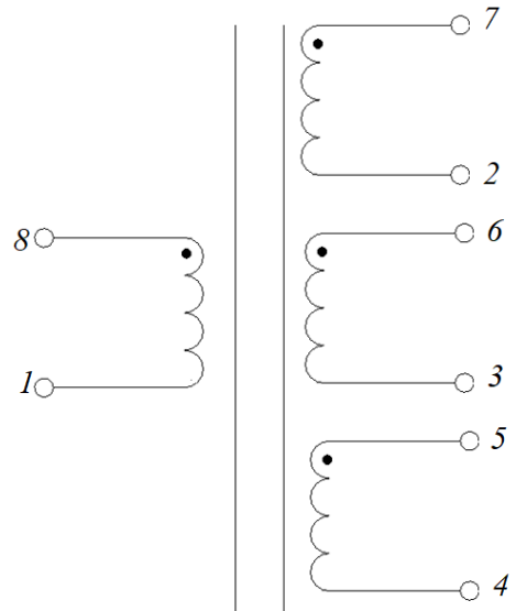
Электрическая схема
