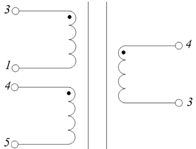
Электрическая схема
