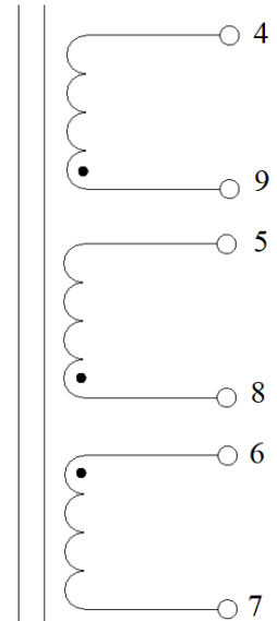
Электрическая схема
