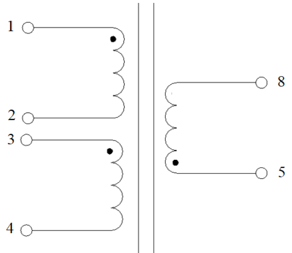
Электрическая схема
