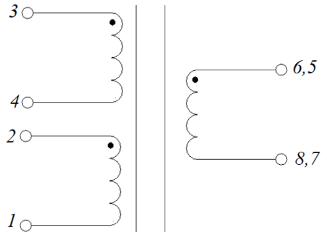
Электрическая схема
