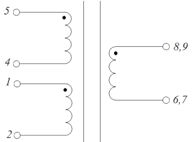
Электрическая схема
