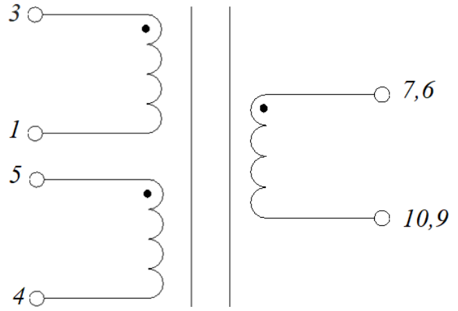
Электрическая схема
