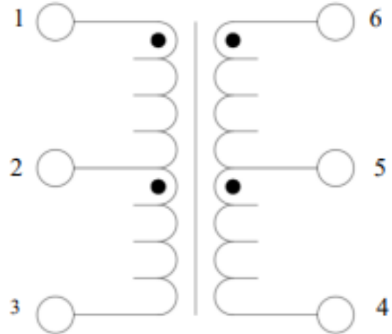
Электрическая схема
