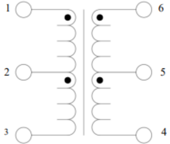
Электрическая схема
