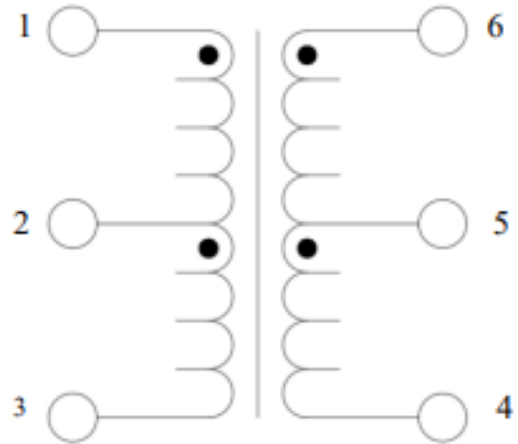
Электрическая схема
