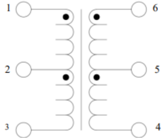
Электрическая схема
