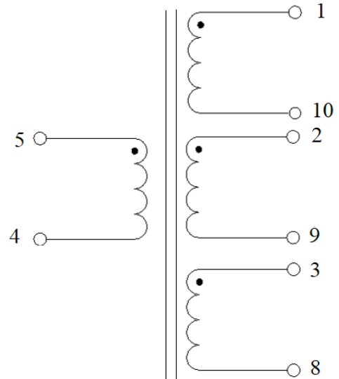
Электрическая схема
