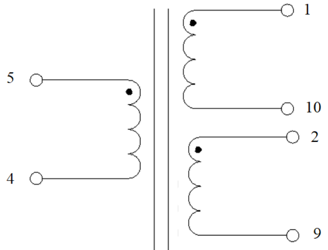
Электрическая схема
