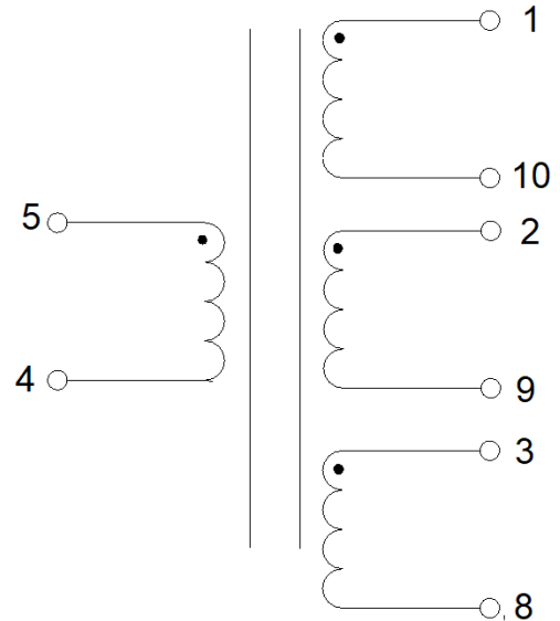
Электрическая схема
