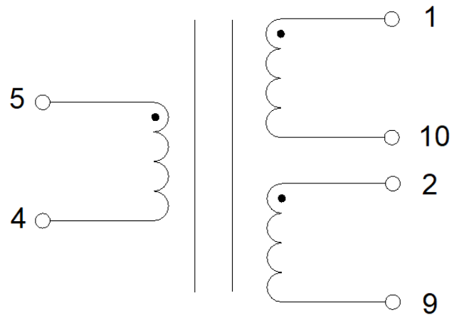
Электрическая схема
