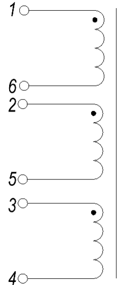
Электрическая схема
