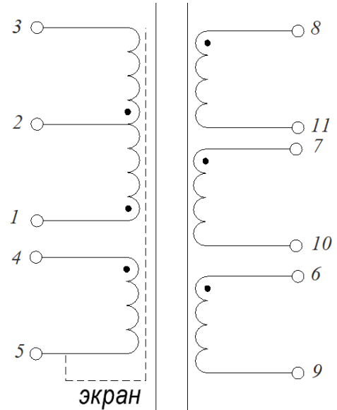
Электрическая схема
