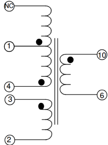
Электрическая схема
