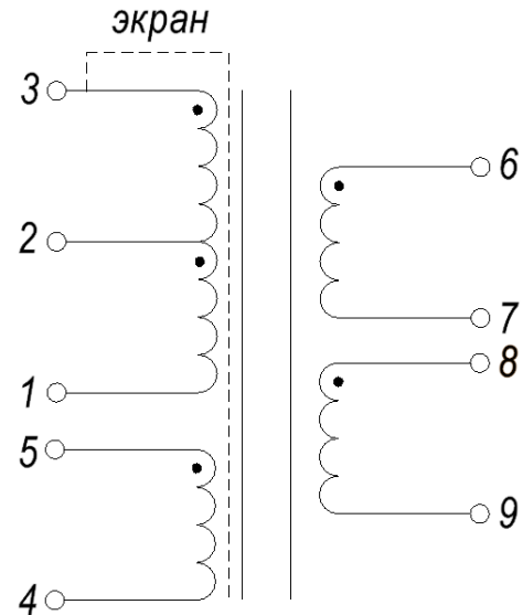
Электрическая схема
