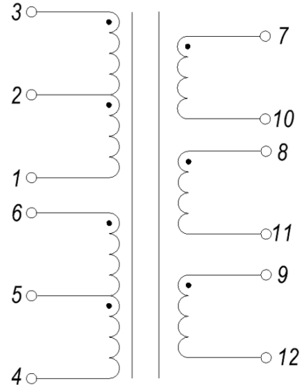
Электрическая схема
