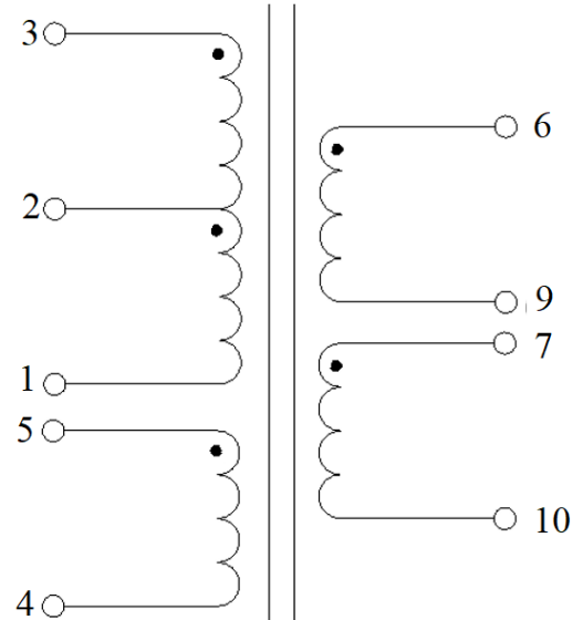
Электрическая схема
