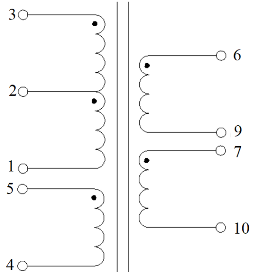
Электрическая схема
