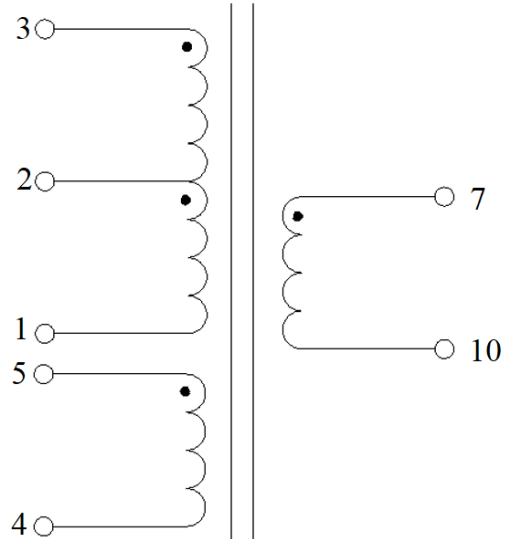
Электрическая схема
