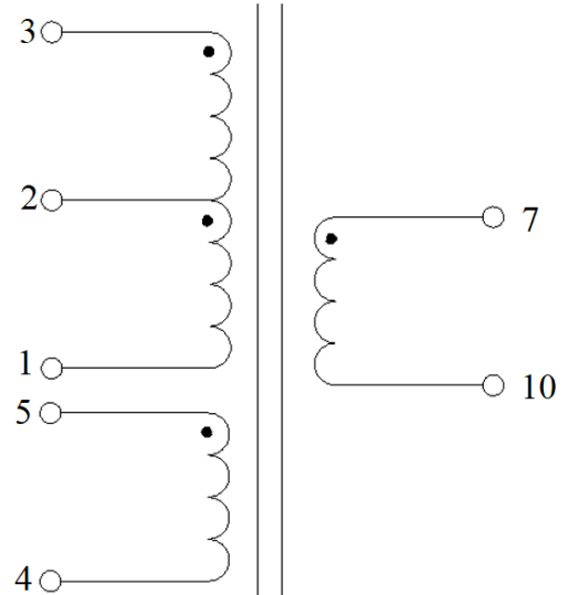
Электрическая схема
