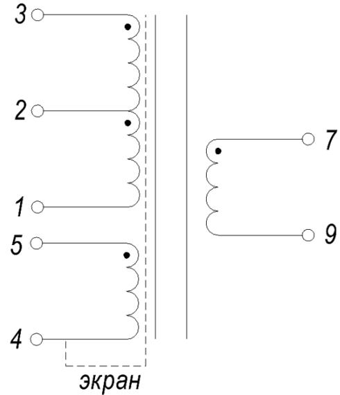
Электрическая схема
