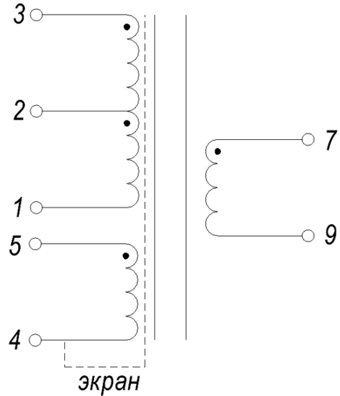
Электрическая схема
