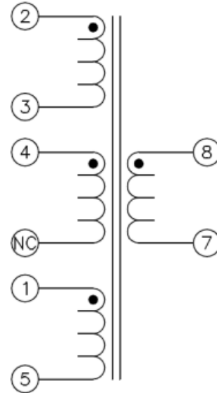
Электрическая схема
