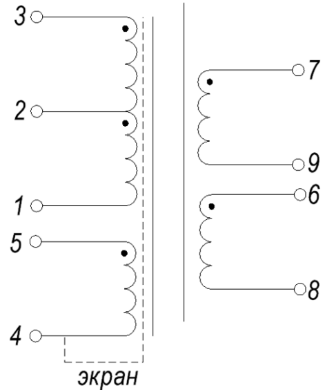
Электрическая схема
