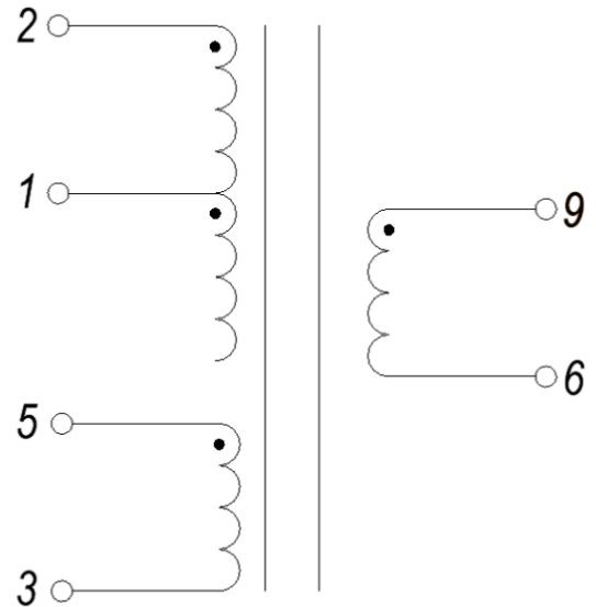
Электрическая схема
