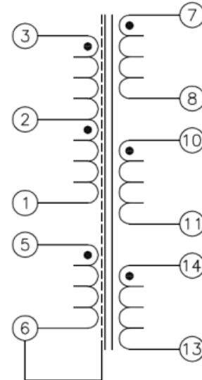
Электрическая схема
