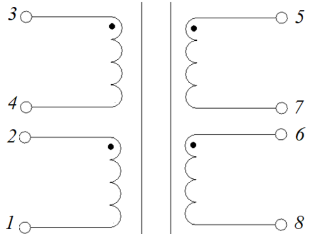
Электрическая схема
