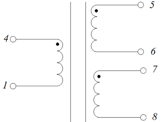
Электрическая схема
