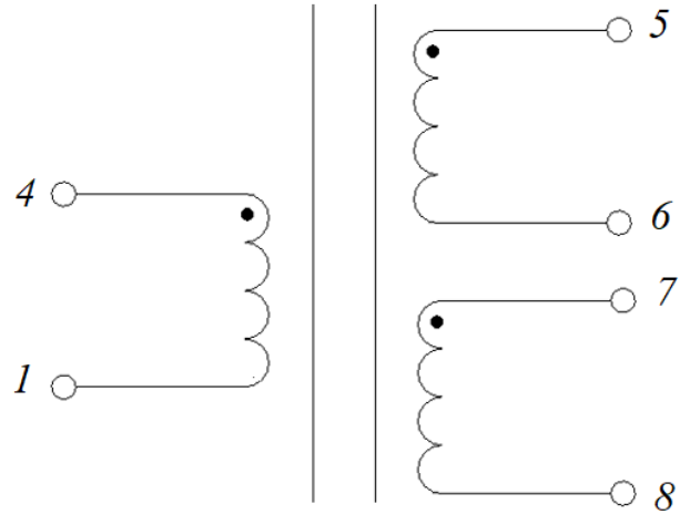
Электрическая схема
