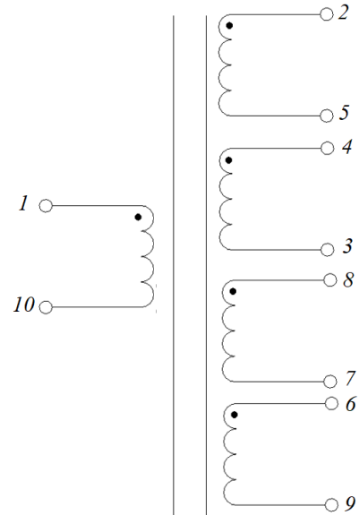
Электрическая схема
