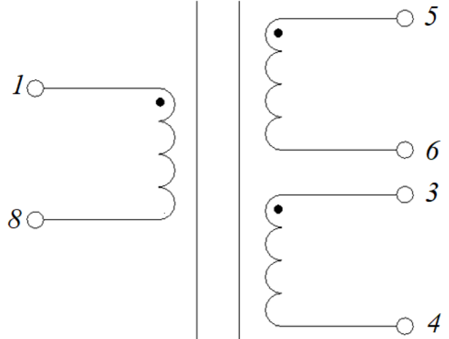
Электрическая схема
