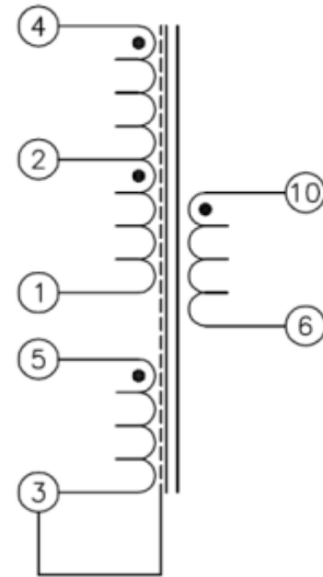
Электрическая схема
