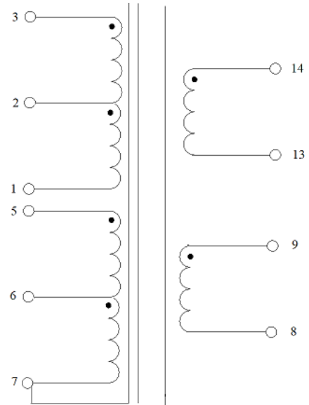
Электрическая схема
