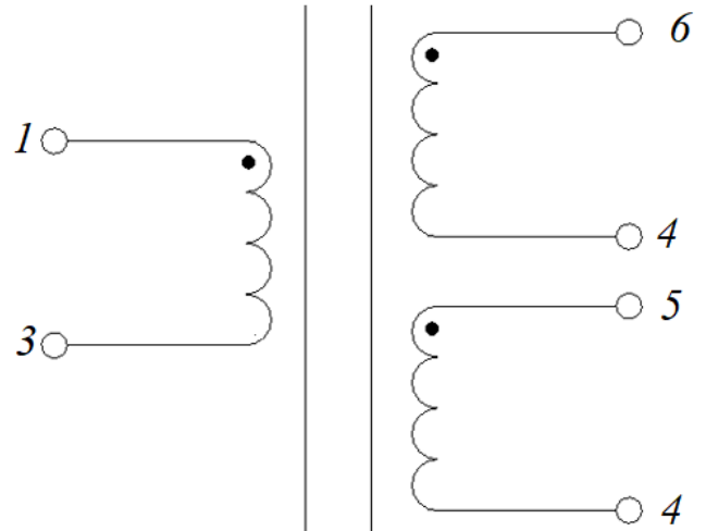
Электрическая схема
