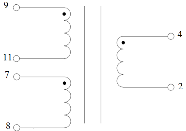
Электрическая схема
