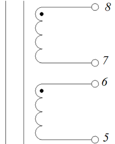
Электрическая схема
