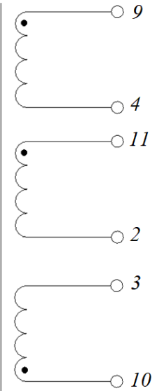
Электрическая схема
