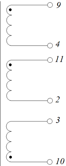
Электрическая схема
