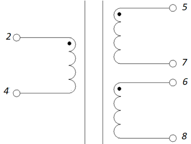
Электрическая схема
