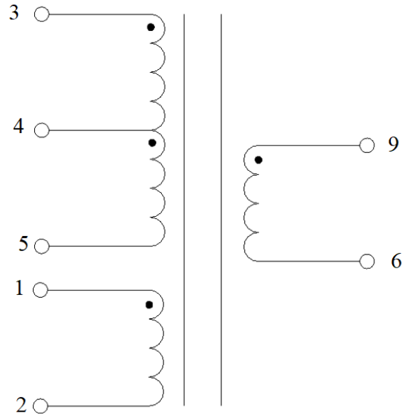
Электрическая схема
