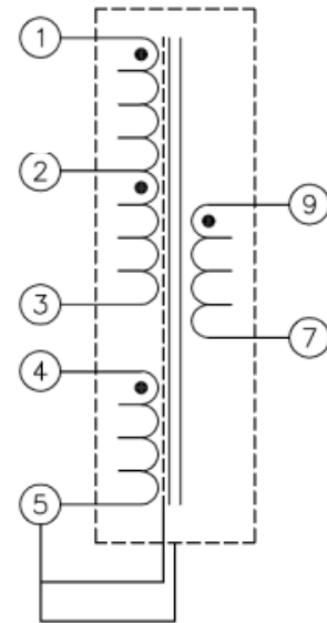
Электрическая схема
