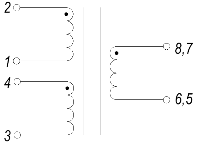
Электрическая схема
