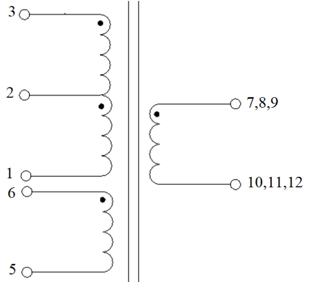
Электрическая схема
