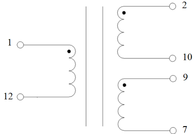
Электрическая схема
